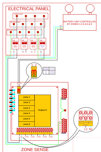
ZNSC2-6Z-10ACGY10
