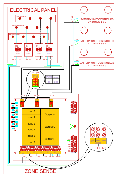
ZNSC2-6Z-30ACGY04
