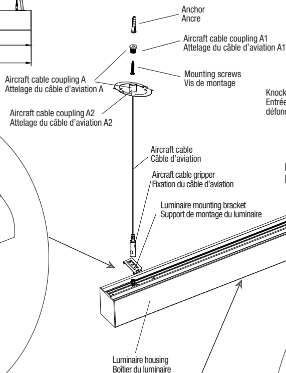
Detail D Détail D
