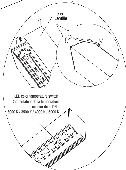
Detail A Détail A
