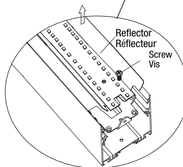
Detail B Détail B
