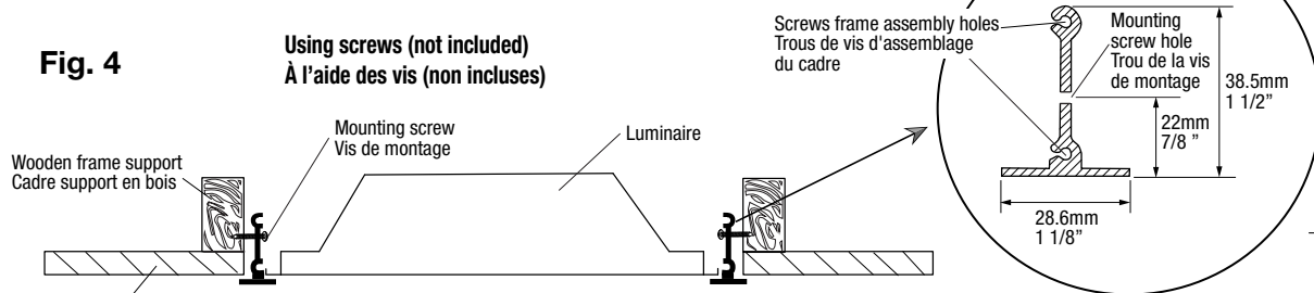
METALLIC FRAME SECTION DETAIL DÉTAIL DE LA SECTION DU CADRE METALLIQUE
